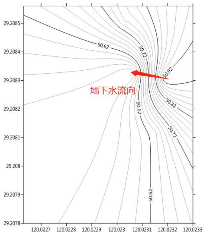
图 2.5-3 本地块所在区域地下水流向等值线图
