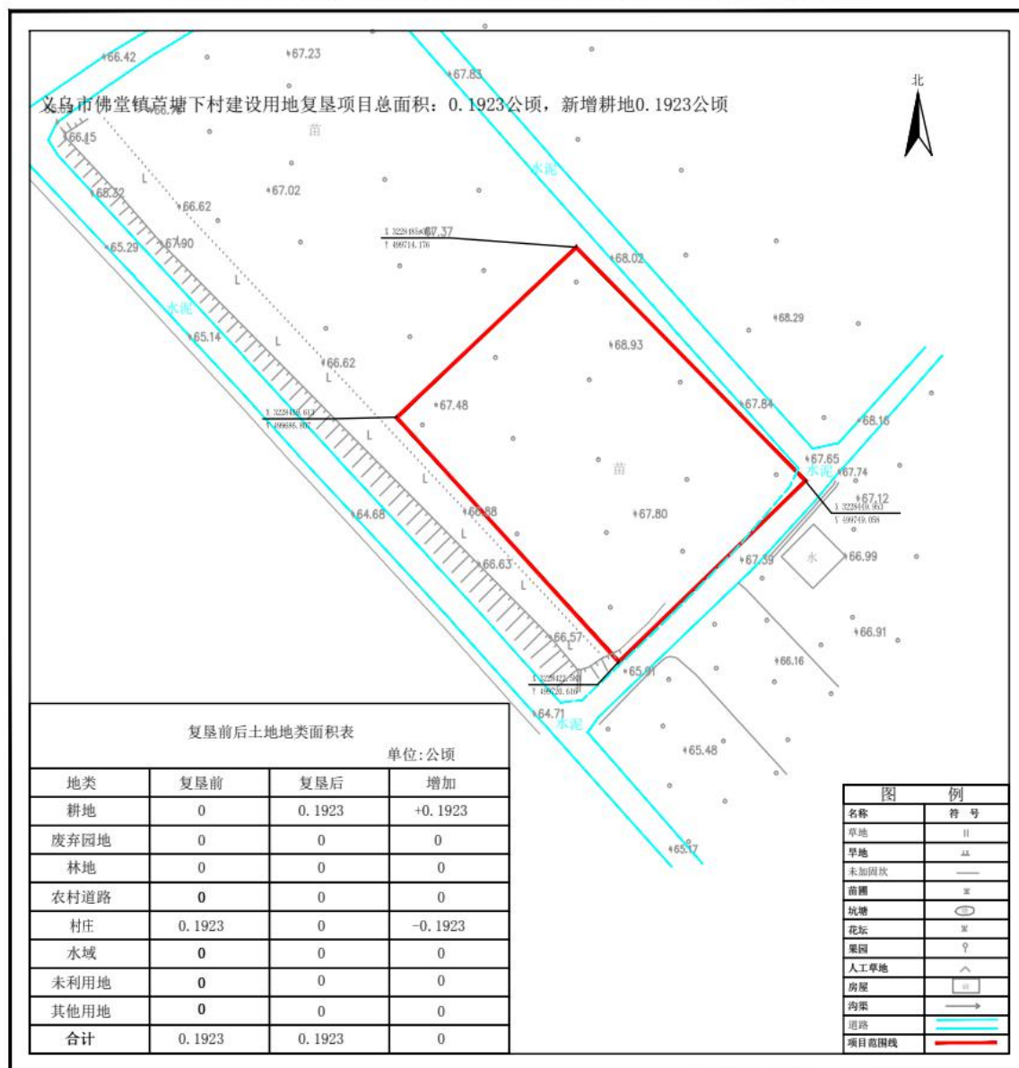
义乌市佛堂镇芦塘下村建设用地复垦项目（2019）竣工图
