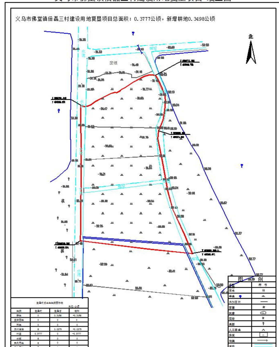
图 2.2-1 调查范围（竣工图）
